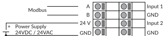
Kuva 2a - Kytkentäkaavio
