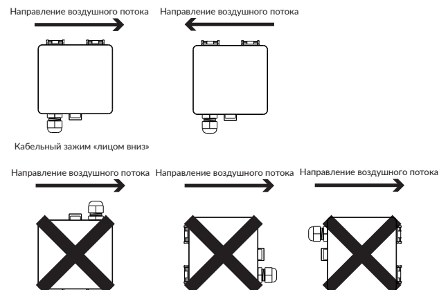
Рисунок 1c - Направление монтажа
