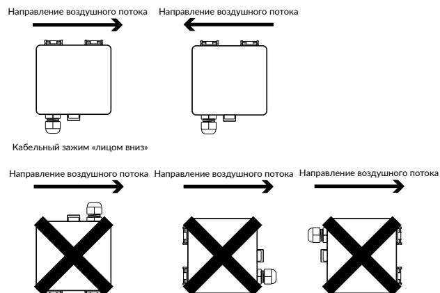
Рисунок 1c - Направление монтажа
