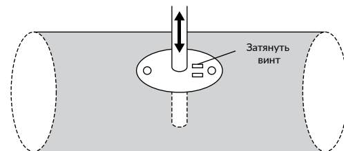
Рисунок 1b - Монтаж датчика во фланце
