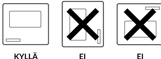
Kuva 1b - Pinta-asennus
