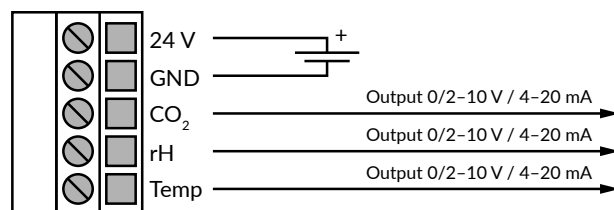
Kuva 2b - KytKentäkaavio: Jännitesyöttö ja ulostulosignaalit
