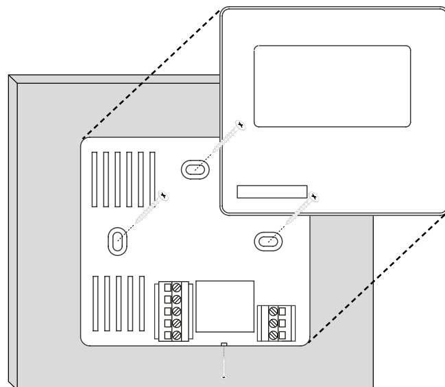
Kuva 1a - Pinta-asennus
