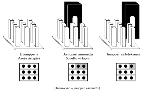
Kuva 3 - Jumperiasetukset
