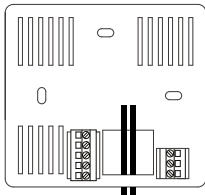
Kuva 2a - Johdotus
