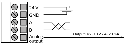
Kuva 2b - Kytkentäkaavio: Jännitesyöttö ja ulostulosignaalit
