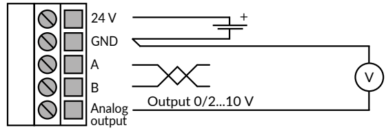
Kuva 2c - Kytkentäkaavio: Ylimääräinen maajohtin
