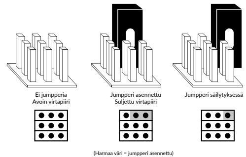
Kuva 3 - Jumpperiasetukset
