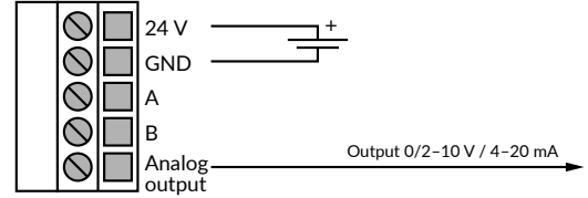
Kuva 2b - KytKentäkaavio: Jännitesyöttö ja ulostulosignaalit
