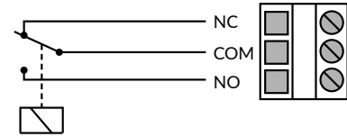
Kuva 2d - KytKentäkaavio: Rele
