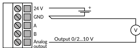
Рисунок 2с - Монтажная электросхема: дополнительный заземленный кабель
