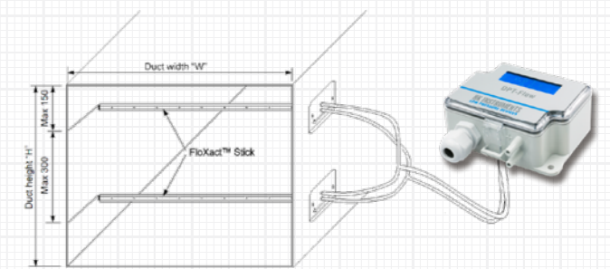
Figura 2. Montaje de FloXact™-L.
